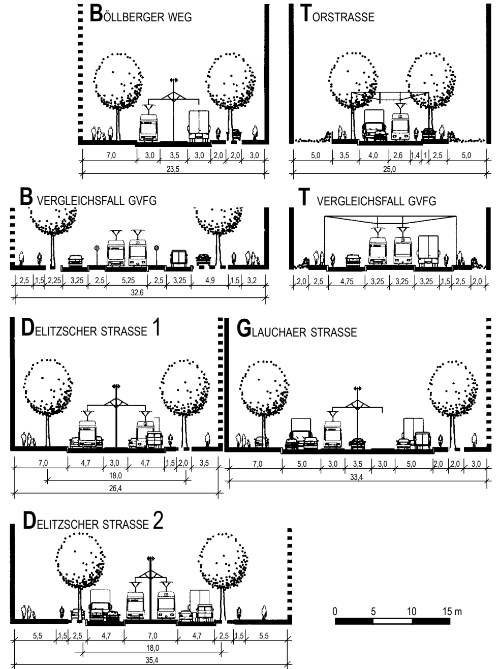
Abb. 2: PLANUNGSBEISPIELE HALLE/SAALE - QUERSCHNITTE
