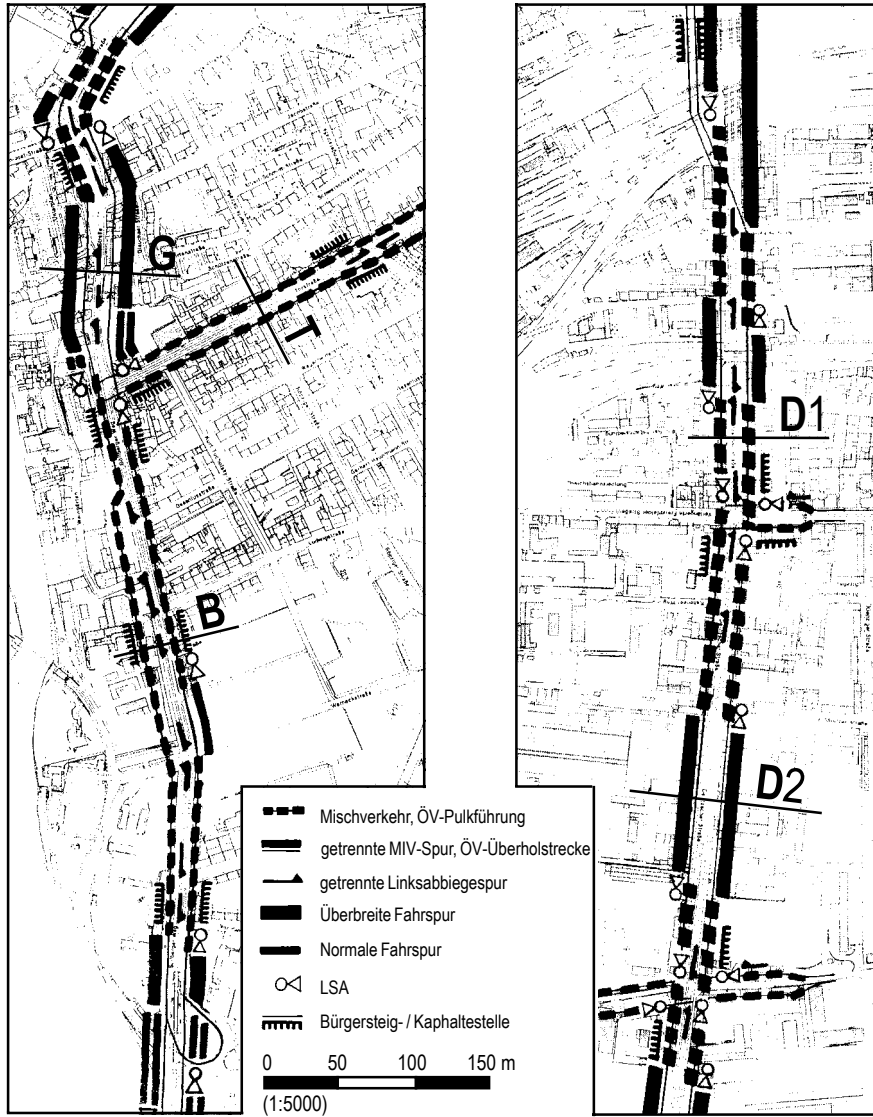
Abb. 1: PLANUNGSBEISPIELE HALLE/SAALE: DIFFERENZIERUNG STRASSENABSCHNITTE
